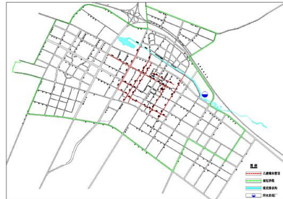
图 7-2 城区现状雨水管网分布图
