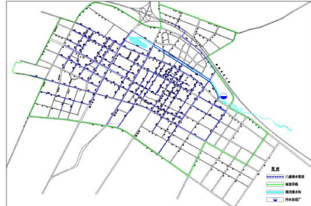
图 7-1 城区现状排水管网分布图
